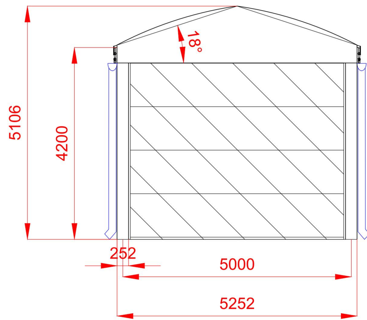
Elevation B
