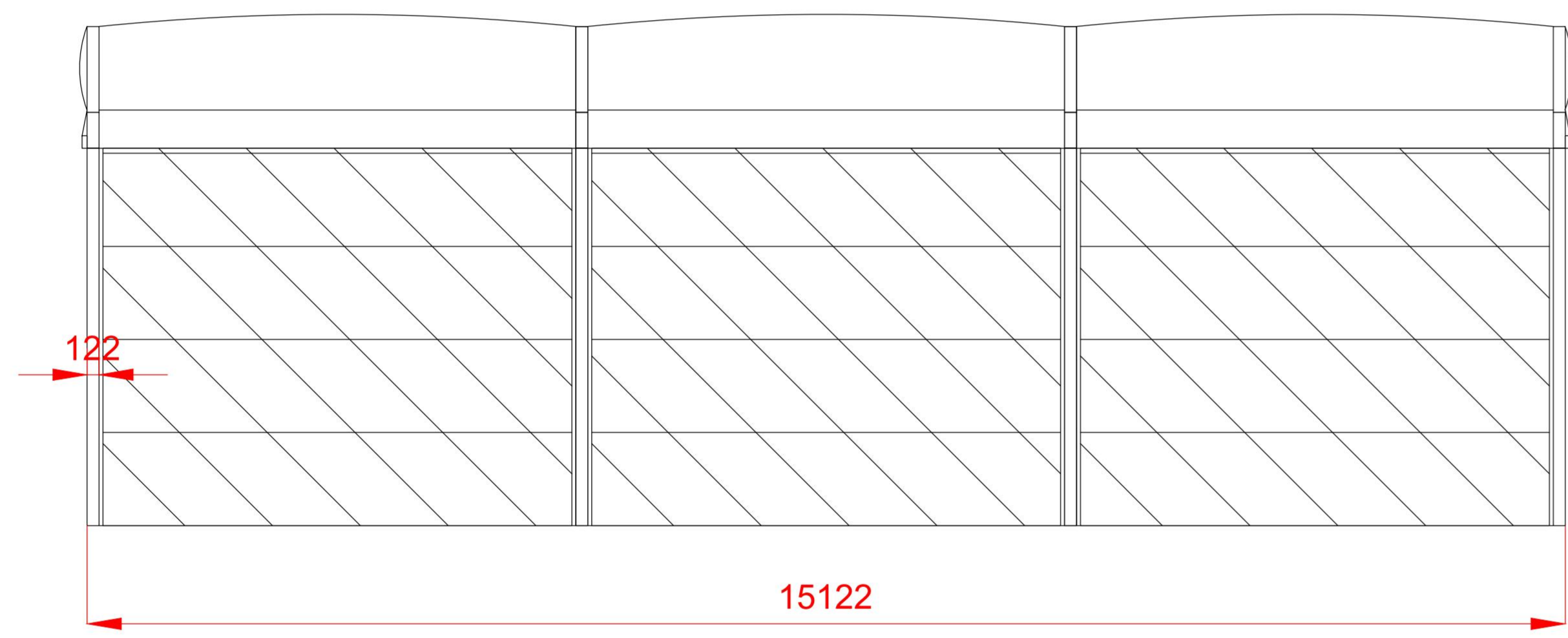
Elevation A
