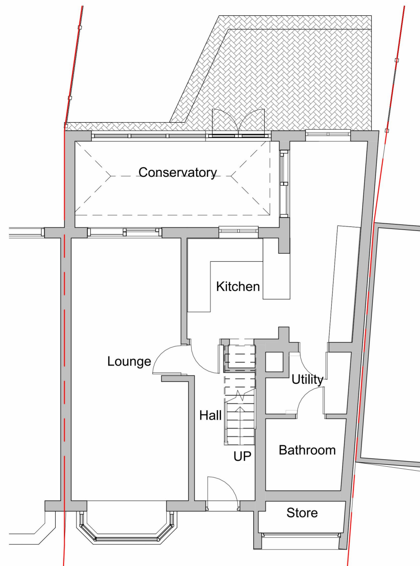
1 _Ground Floor Existing Plan_ 1 : 100
