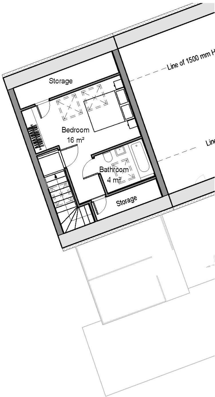
2 LEVEL 03 - Loft 1 : 100
